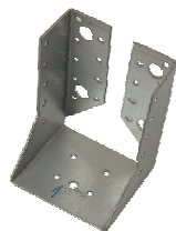
art. 4596 Nosač grede unutrašnji 80 mm 4596.1 Nosač grede unutrašnji 100*140*75 mm WBZ24 4596.2 Nosač grede unutrašnji 120*160*80 mm WBZ25
